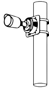
連接桿安裝
